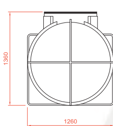
END ELEVATION
